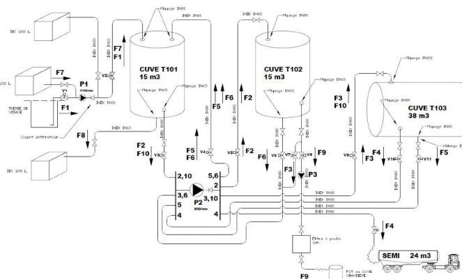
TRIAlP 73000 CHAMBERY SCHEMA DE PRINCIPE TRANSFERT HUILE
